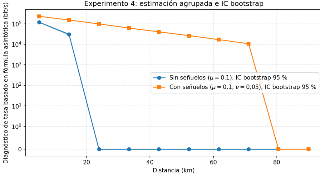
Figura 7: Diagnósticos con conteos agrupados y fórmulas asintóticas, ambos con \mu = 0,1 . Las bandas son IC bootstrap pareados del 95 %; la configuración señuelo usa \nu = 0,05 y Y_0 = 2,40 \times 10^{-7} .
