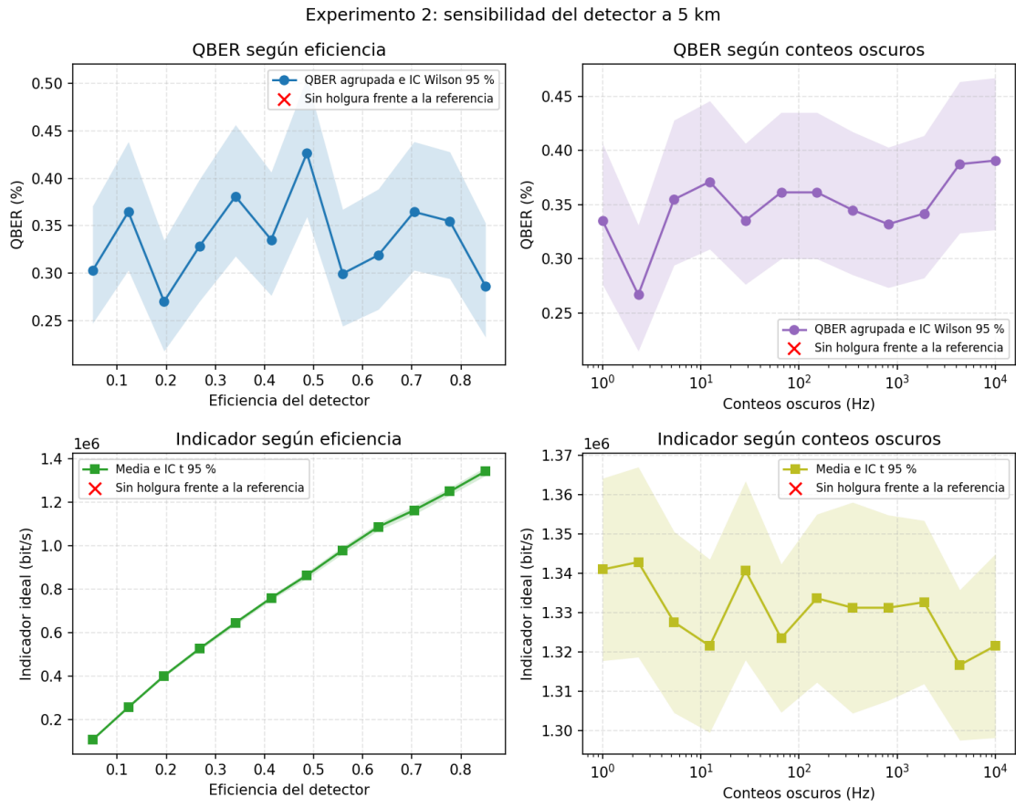
Figura 5: QBER e indicador ideal frente a eficiencia y conteos oscuros a 5,00 km. Todos los puntos conservan holgura frente a la referencia analítica.
