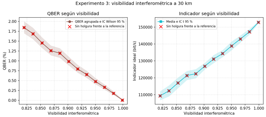
Figura 8.4: Respuesta del modelo a la visibilidad a 30 km. Las cruces señalan ausencia de holgura frente a la referencia analítica de tasa.
