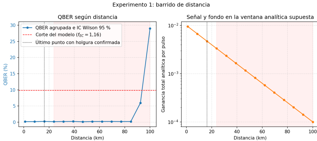
Figura 8.1: QBER agrupada con IC de Wilson del 95 % y ganancia total analítica. La zona roja comienza donde la tasa tamizada simulada deja de conservar holgura frente a la referencia.
