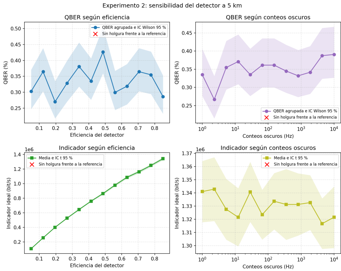
Figura 8.3: QBER e indicador ideal frente a eficiencia y conteos oscuros a 5 km. QBER usa IC de Wilson y el indicador usa IC t entre repeticiones.
