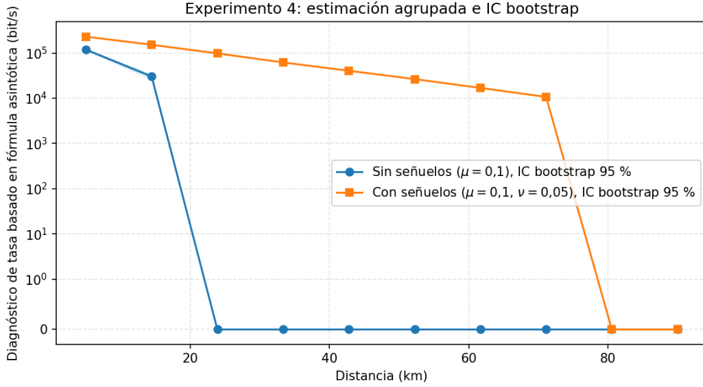
Figura 8.5: Diagnósticos de tasa calculados con conteos agrupados y fórmulas asintóticas, ambos con \mu = 0,1 . Las bandas son IC bootstrap pareados del 95 %; la configuración señuelo usa \nu = 0,05 y Y_0 = 2,40 \times 10^{-7} .
