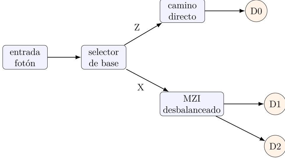
Figura 2.3: Receptor time-bin conceptual: medición directa para base Z y dos puertos monitoreados en el Mach–Zehnder de la base X. Sólo la ventana central de D1/D2 forma bits X.
