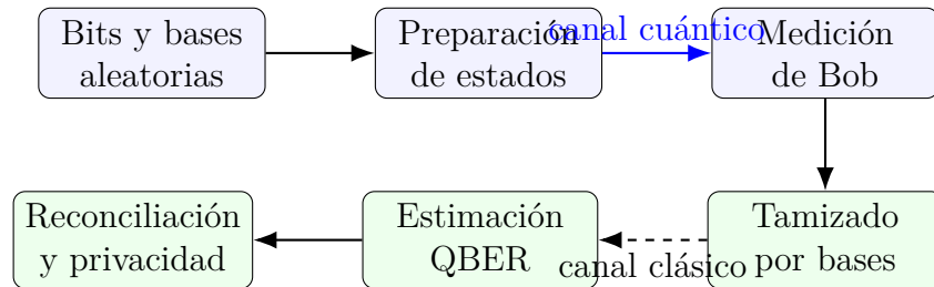
Figura 2.1: Secuencia funcional de BB84 desde preparación hasta postprocesamiento.
