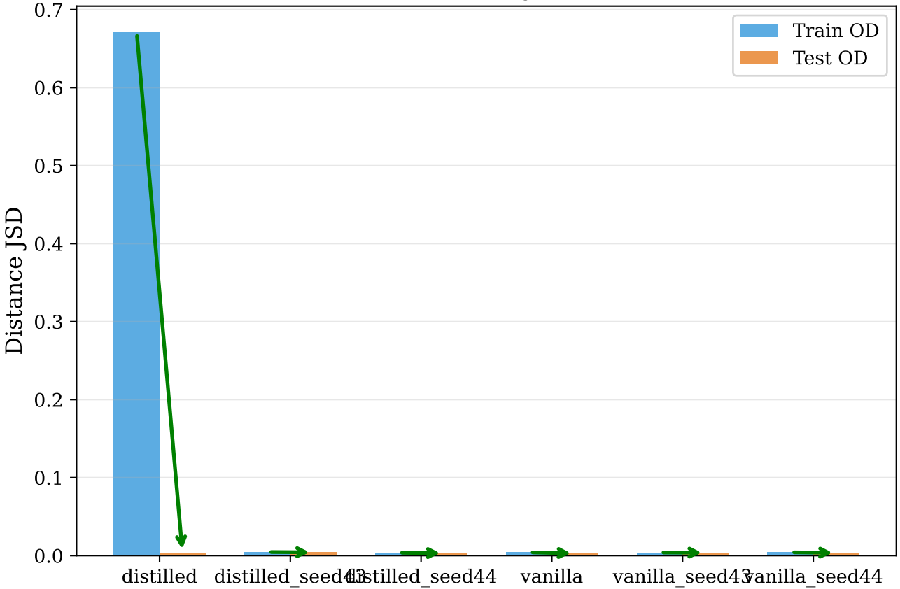
Distance JSD
