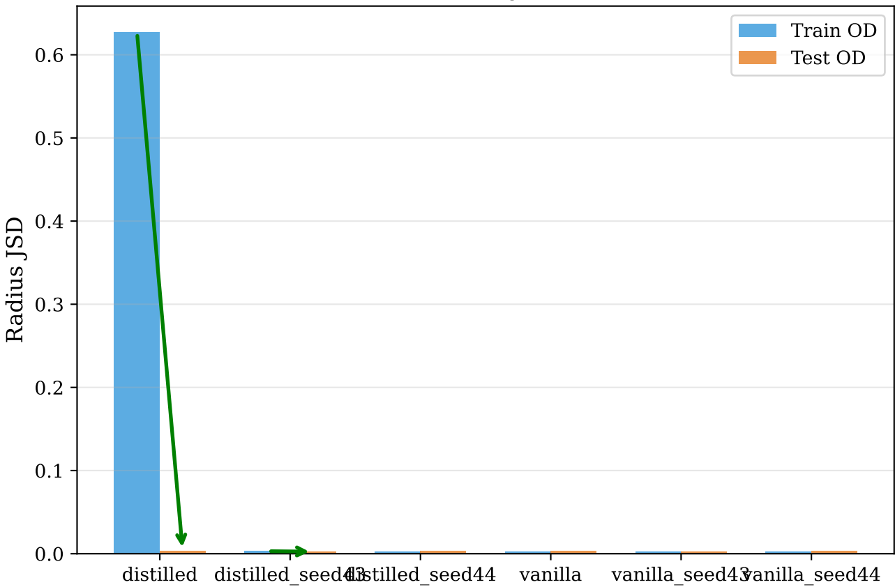
Radius JSD
