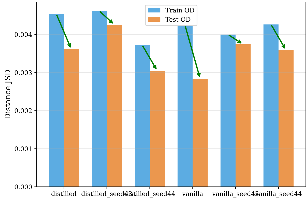
Distance JSD
