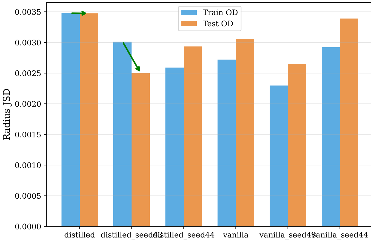
Radius JSD
