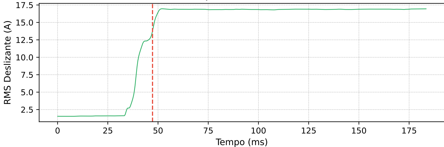
RMS Deslizante (janela = 1 ciclo = 128 amostras)
