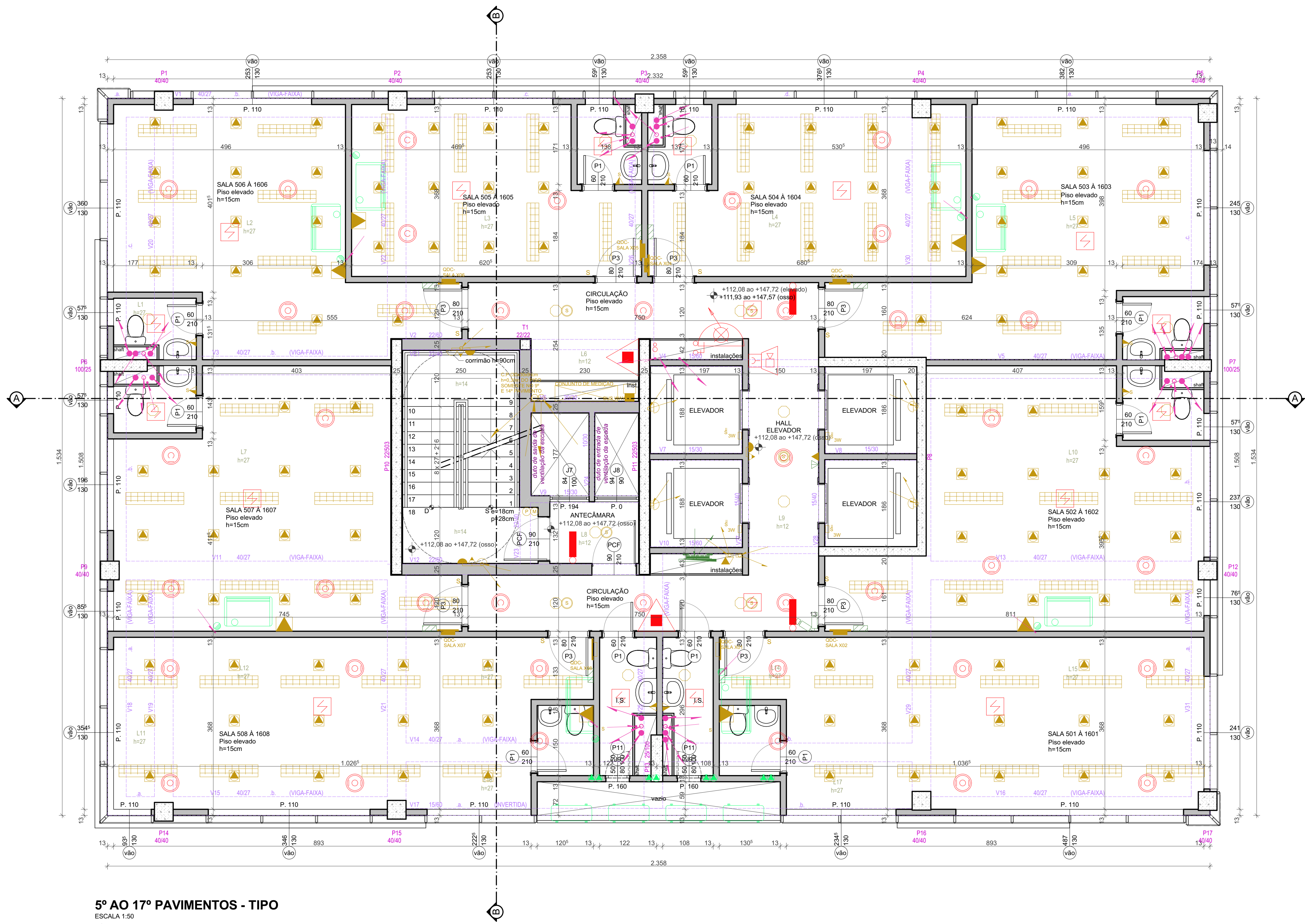
5º AO 17º PAVIMENTOS - TIPO ESCALA 1:50
