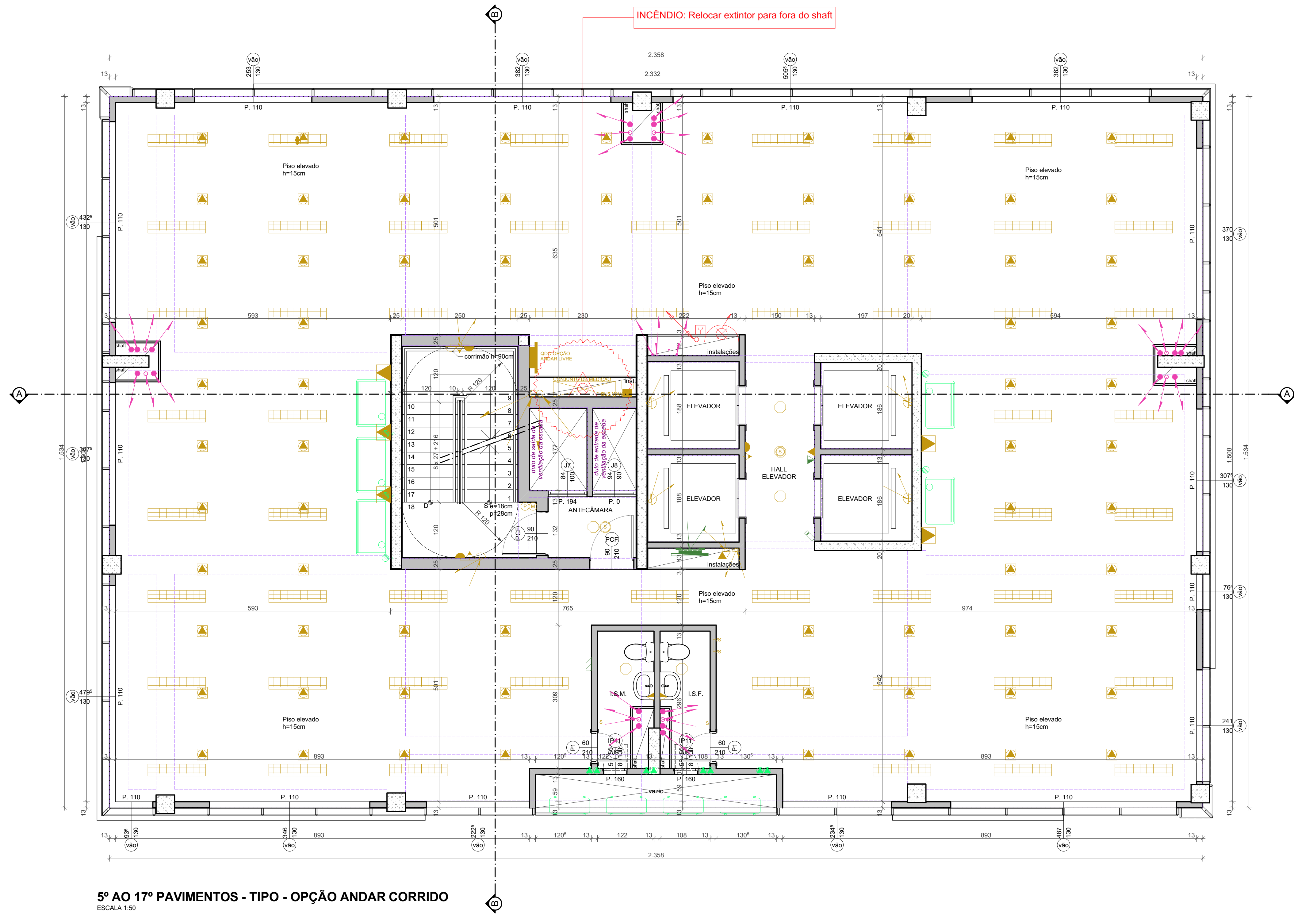
5º AO 17º PAVIMENTOS - TIPO - OPÇÃO ANDAR CORRIDO ESCALA 1:50
