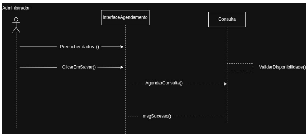
Figura 3 — Diagrama de Sequência: fluxo de agendamento
