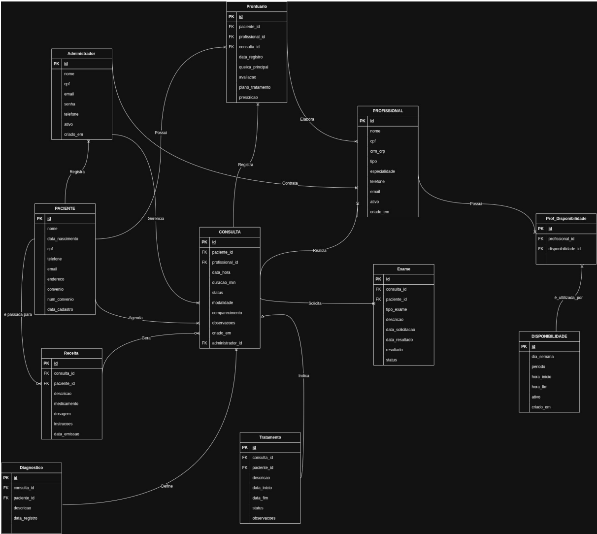
Figura 4 — Diagrama Entidade-Relacionamento do sistema NeuroSpectrum
