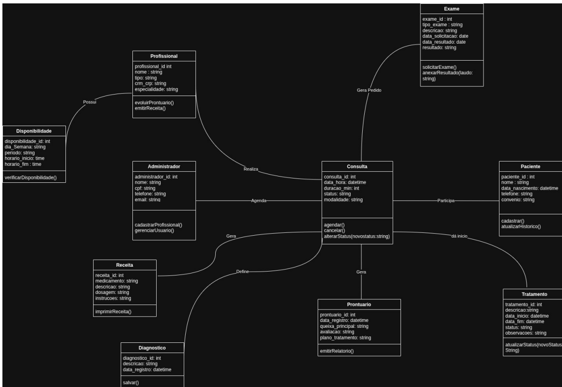
Figura 1 — Diagrama de Classes UML do sistema NeuroSpectrum
