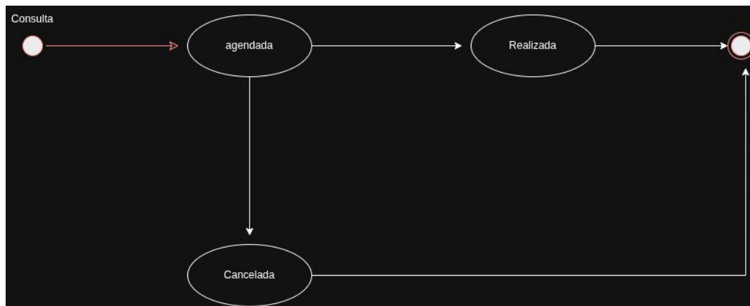
Figura 2 — Diagrama de Estados: ciclo de vida da Consulta
