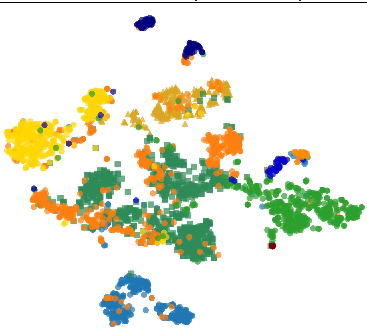
True Classes (Wo Anom.)
