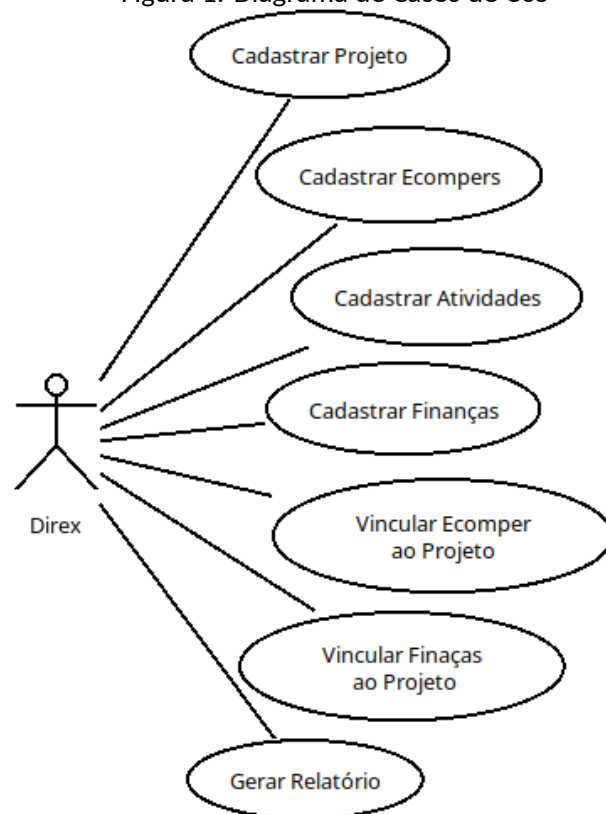
Figura 1: Diagrama de Casos de Uso
