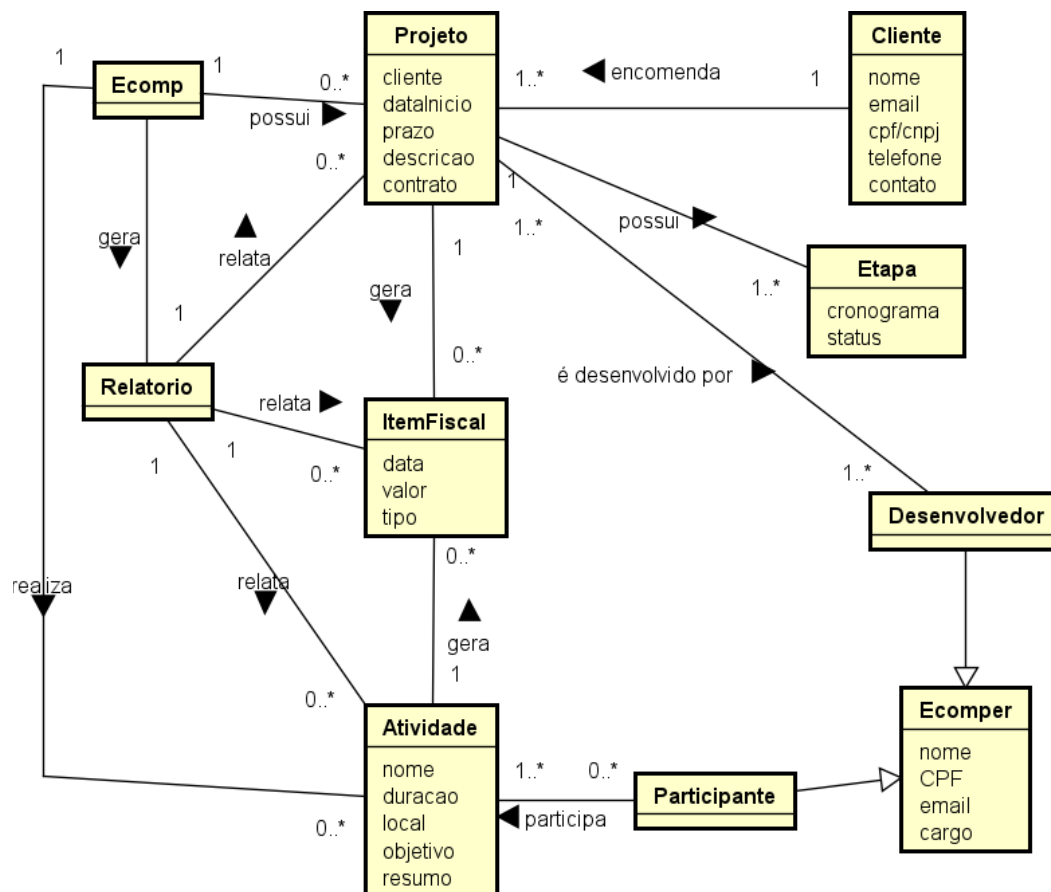
Figura 2: Diagrama classes conceituais
