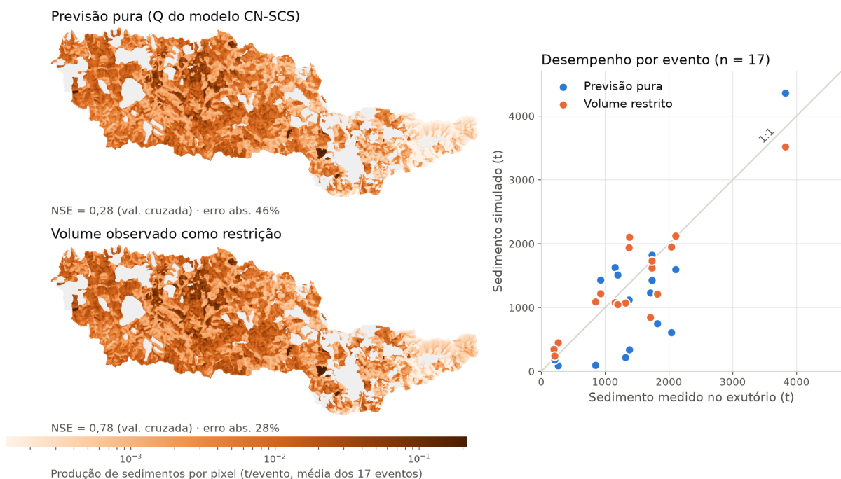
Figura 1 – Mapa de produção de sedimentos nas duas configurações e desempenho por evento
