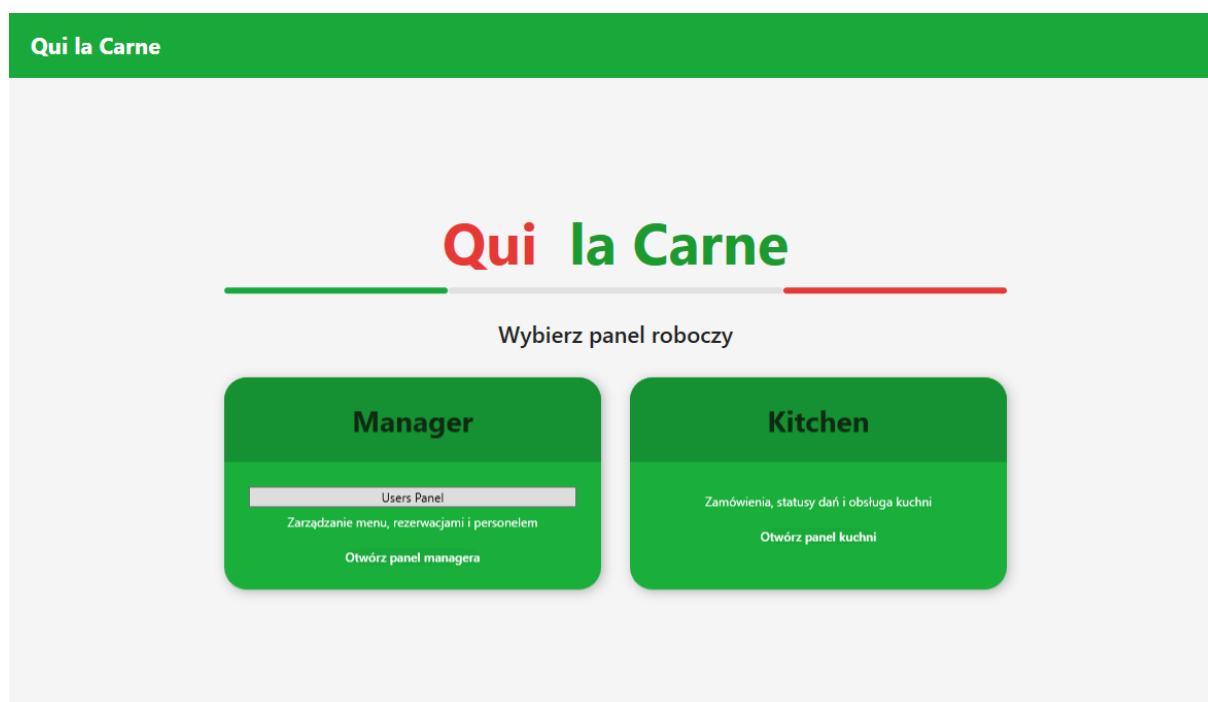
Rysunek 12: Przykładowy widok aplikacji desktop cz.2.
