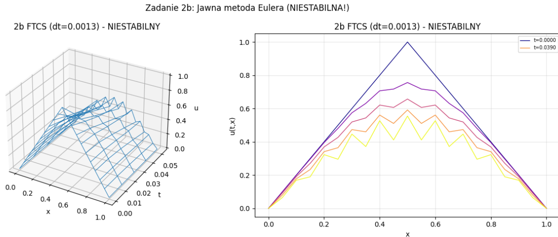
Wykres 6: Numeryczna eksplozja rozwiązania przy \Delta t = 0,0013 ( r = 0,52 > 0,5 ). Warunek stabilności von Neumanna nie jest spełniony.
