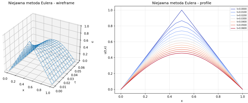
Wykres 7: Stabilne rozwiązanie metodą niejawną BTCS przy dużym kroku czasowym ( \Delta t = 0,005 , r = 2,0 ).
