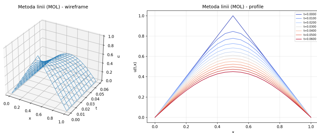
Wykres 9: Rozwiązanie równania ciepła metodą linii (MOL) przy użyciu solwera Radau.
