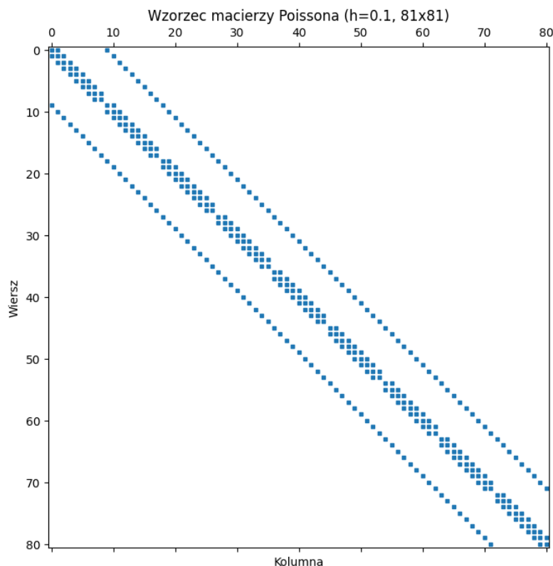
Wykres 1: Wzorzec niezerowych elementów macierzy Poissona ( h = 0,1 , układ 81 \times 81 ).
