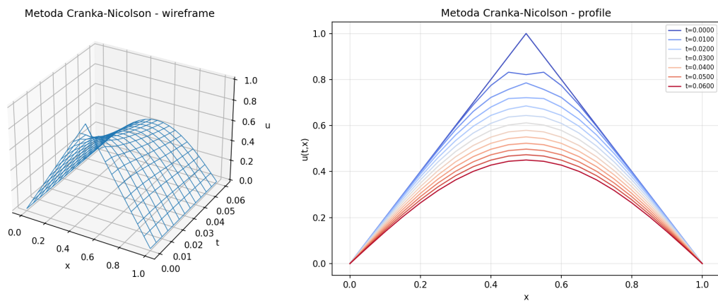
Wykres 8: Rozwiązanie równania ciepła metodą Cranka-Nicolson ( \Delta t = 0,005 , r = 2,0 ).
