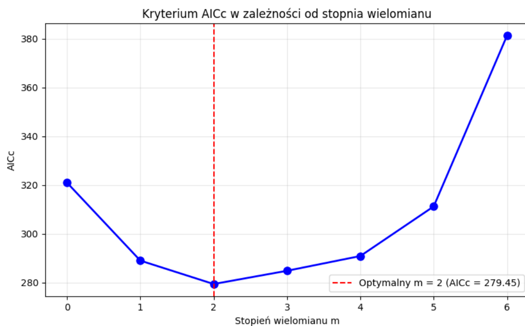
Wykres 2: Wartości AICc dla wielomianów stopnia m = 0 \dots 6 .
