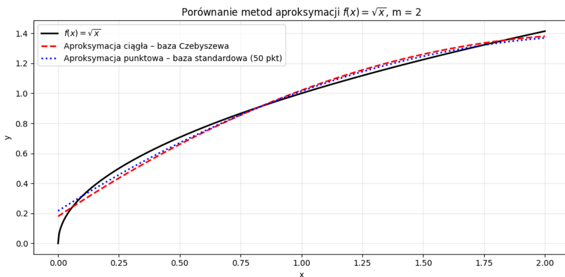
Wykres 4: Porównanie aproksymacji Czebyszewa z klasycznym wielomianem MNK stopnia 2 oraz wykresy błędów obu metod.
