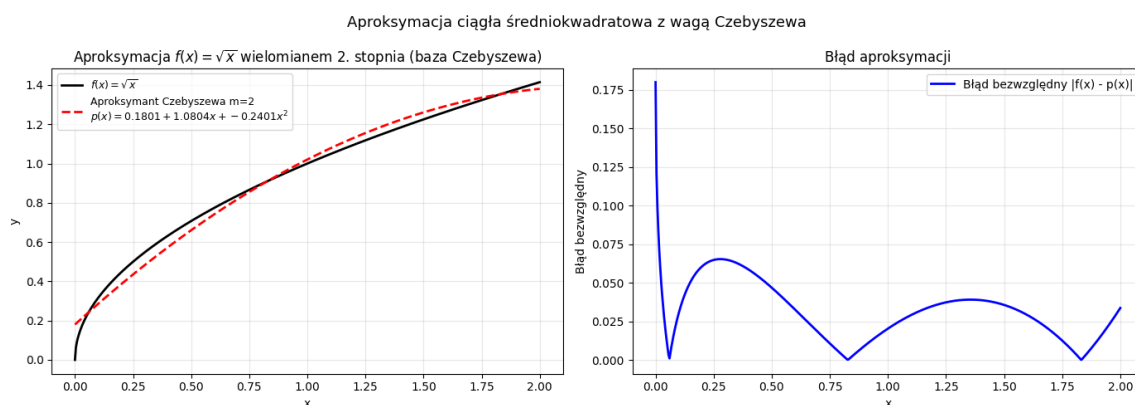
Wykres 3: Aproxymacja f(x) = \sqrt{x} wielomianem 2. stopnia (baza Czebyszewa) i wykres błędu bezwzględnego.
