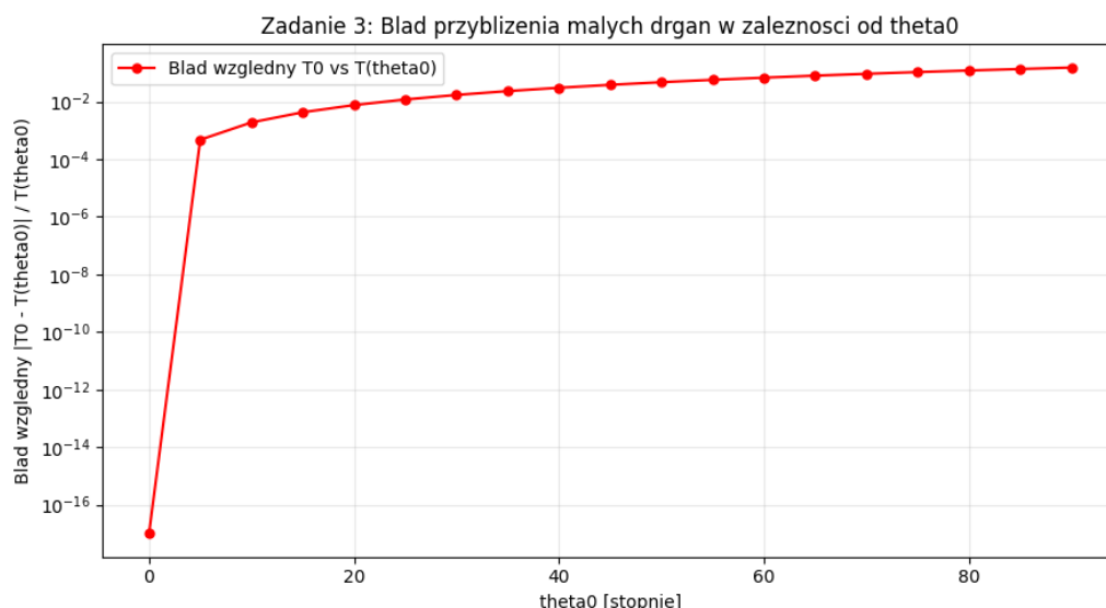
Wykres 4: Błąd względnny okresu T_0 (przybliżenie małych drgań) w zależności od amplitudy \theta_0 .
