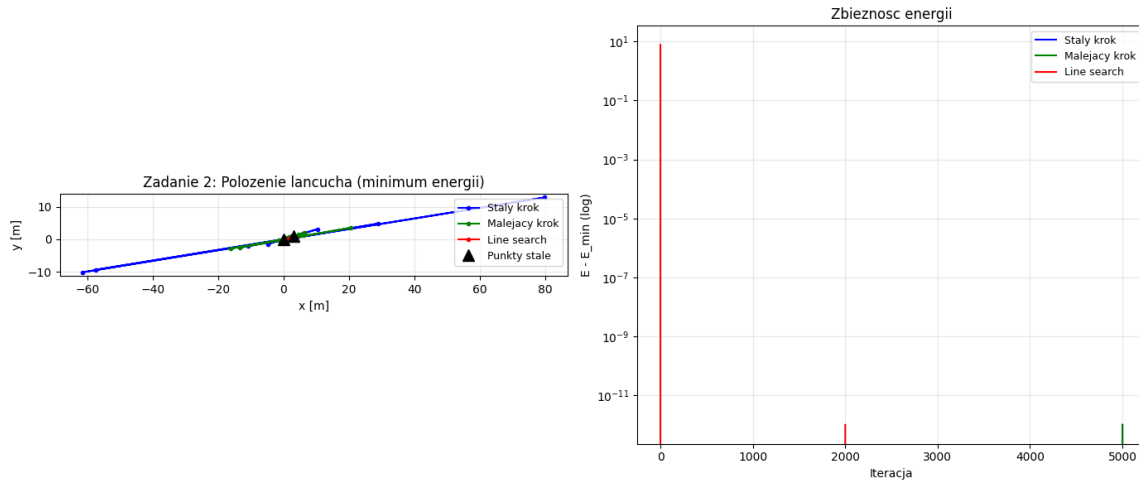
Wykres 3: Położenie mas łańcucha po optymalizacji (po lewej) oraz wykres zbieżności energii w skali logarytmicznej (po prawej) dla trzech badanych wariantów.
