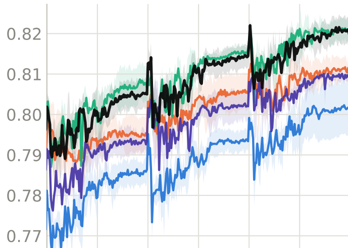
Sparsity 0.7
