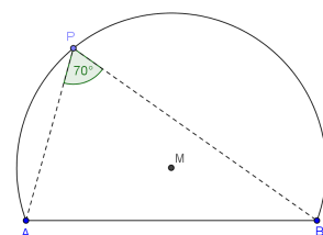
Fasskreisbogen
