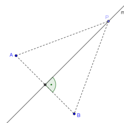
Mittelsenkrechte
