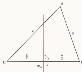
Mittelsenkrechte
