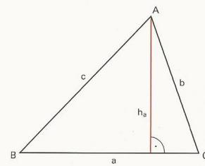
Höhe
