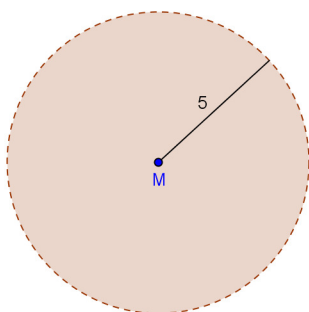
Kreis
