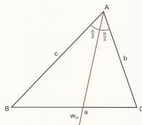
Winkelhalbierende
