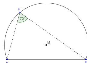
Fasskreisbogen
