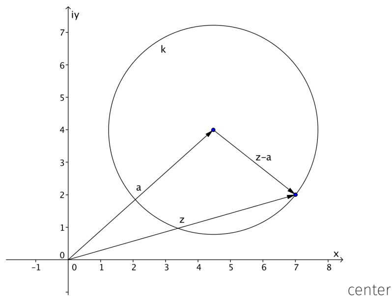
Abb. B.3.: Kreis in der Gaußschen Ebene
