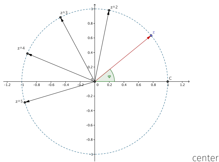
Abb. 4.2.: Die n -te Potenz der komplexen Zahl z geometrisch interpretiert
