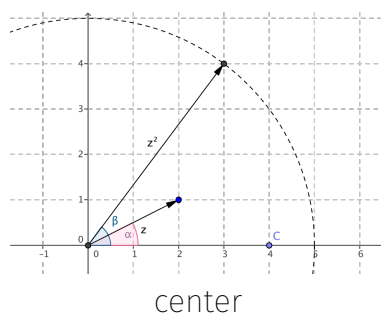
Abb. 4.1.: Quadrieren einer komplexen Zahl z geometrisch interpretiert
