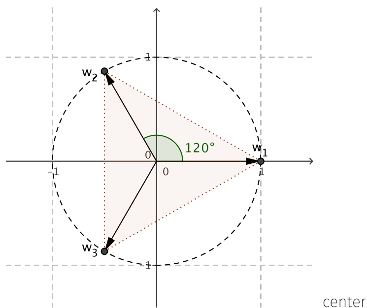
Abb. 4.3.: Die drei dritten „Wurzeln“ aus 1
