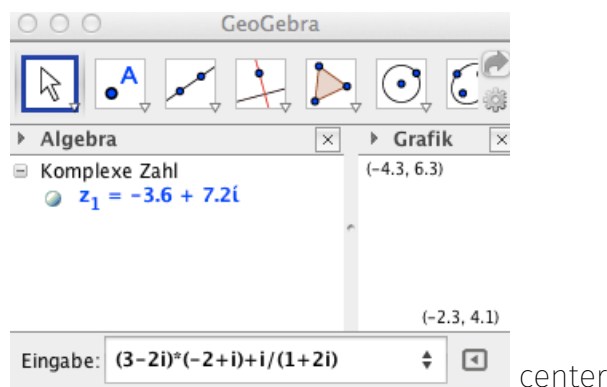
Abb. 3.2.: Rechnen mit komplexen Zahlen in GeoGebra
