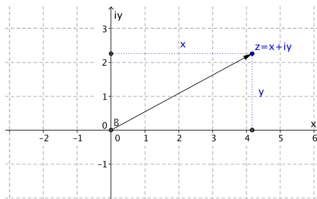
Abb. 3.1.: Komplexe Zahl als Ortsvektor
