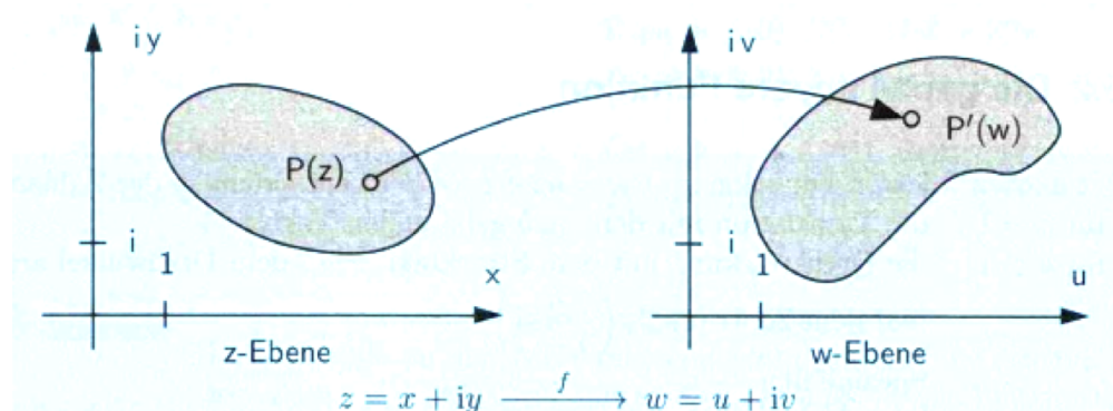
Abb. 1.2.: Visualisierung einer komplexen Funktion \mathbb{C} \rightarrow \mathbb{C}
