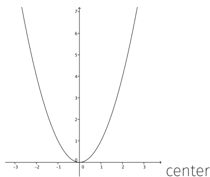
Abb. 1.1.: Graph einer quadratischen Funktion \mathbb{R} \rightarrow \mathbb{R}
