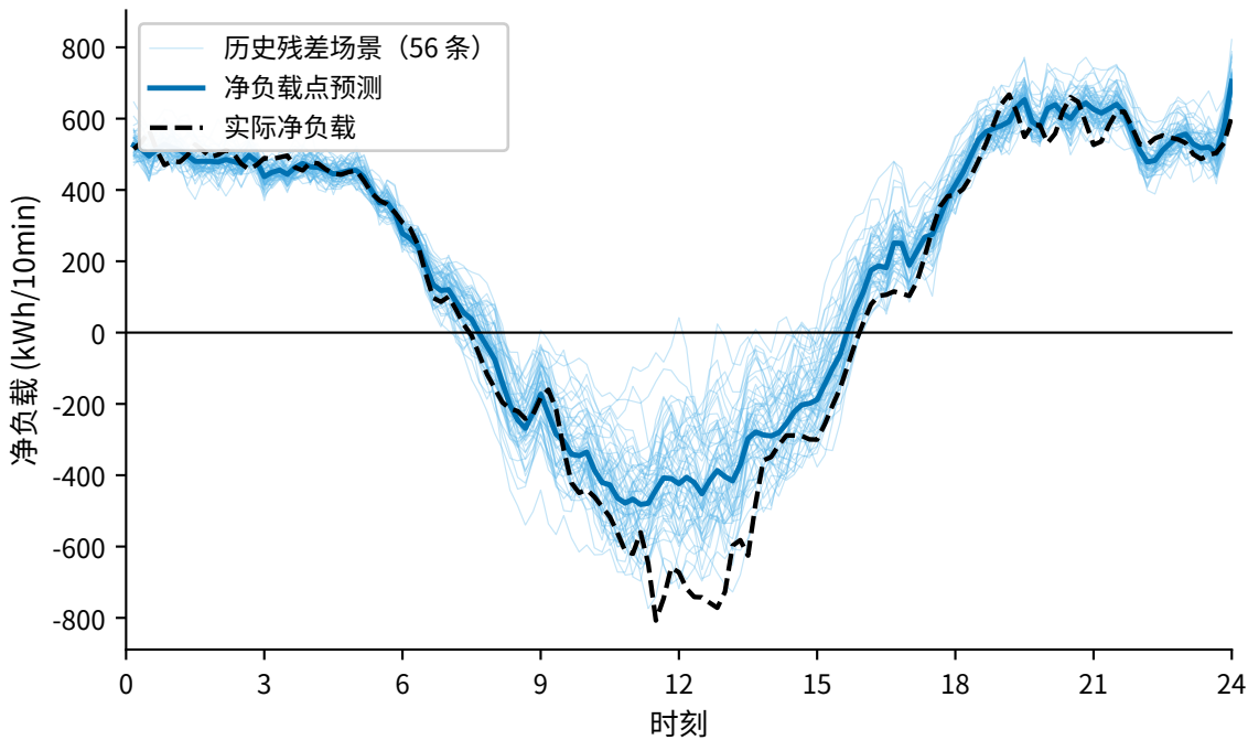
(a) 2025-06-21 净负载预测与场景集
