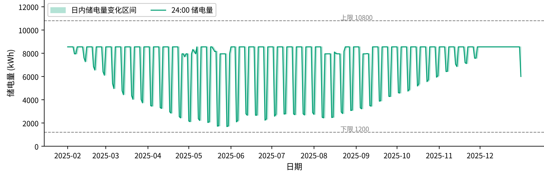
(b) 逐日储电量轨迹
