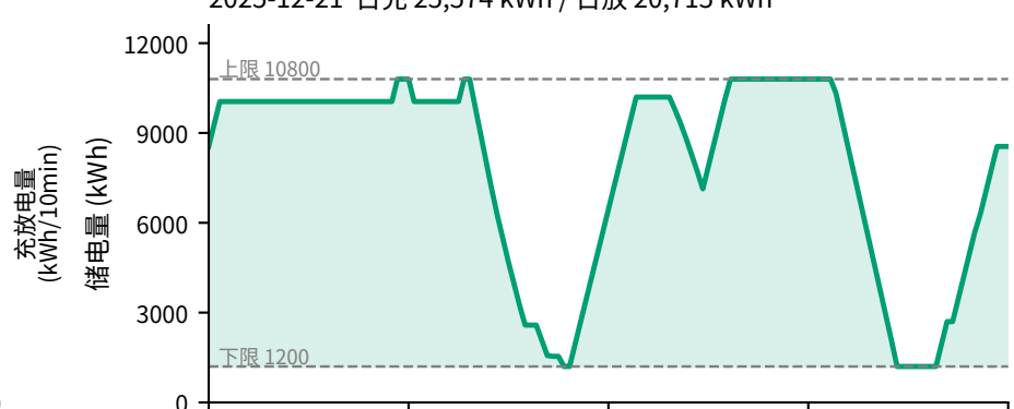
2025-12-21 日充 25,574 kWh / 日放 20,715 kWh
