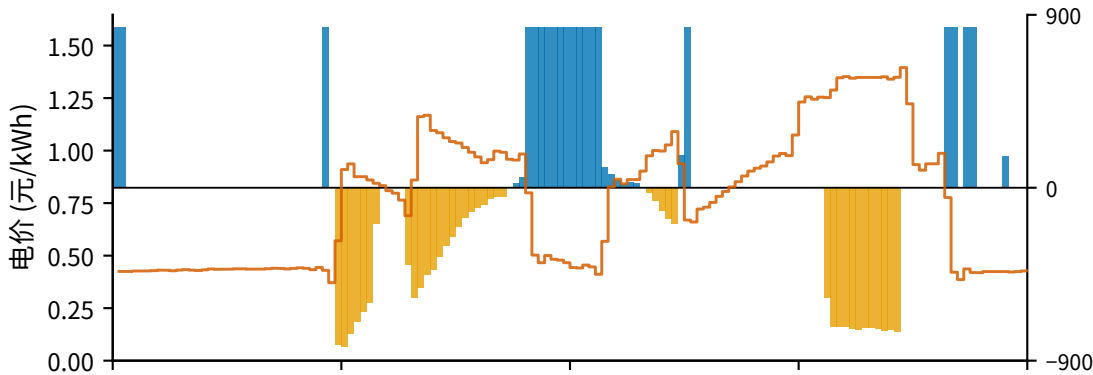
问题2 指定日期的储能充放电与储电量轨迹
