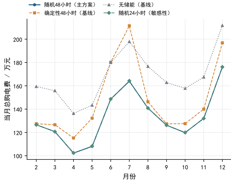
(b) 月度费用变化
