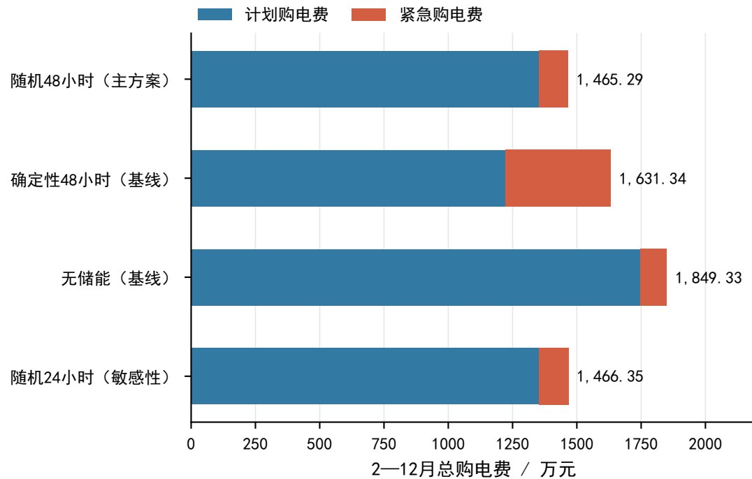
(a) 同期费用及构成
