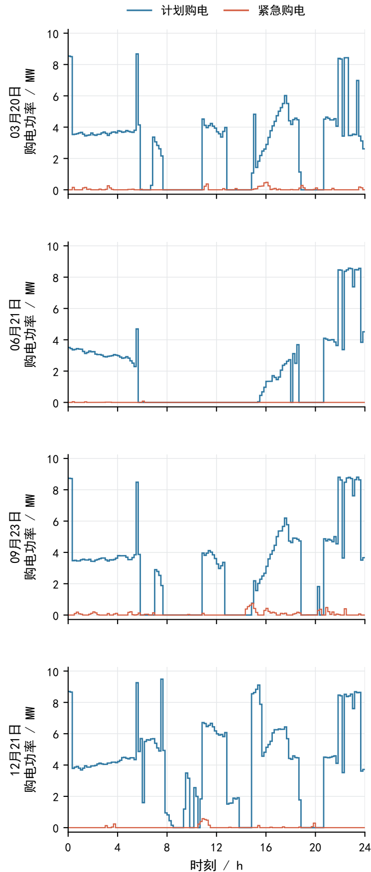
(a) 计划与紧急购电
