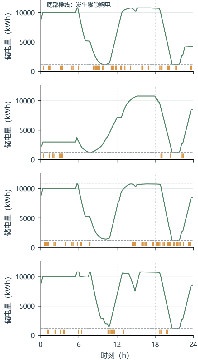
(b) 储能状态与紧急购电时段
