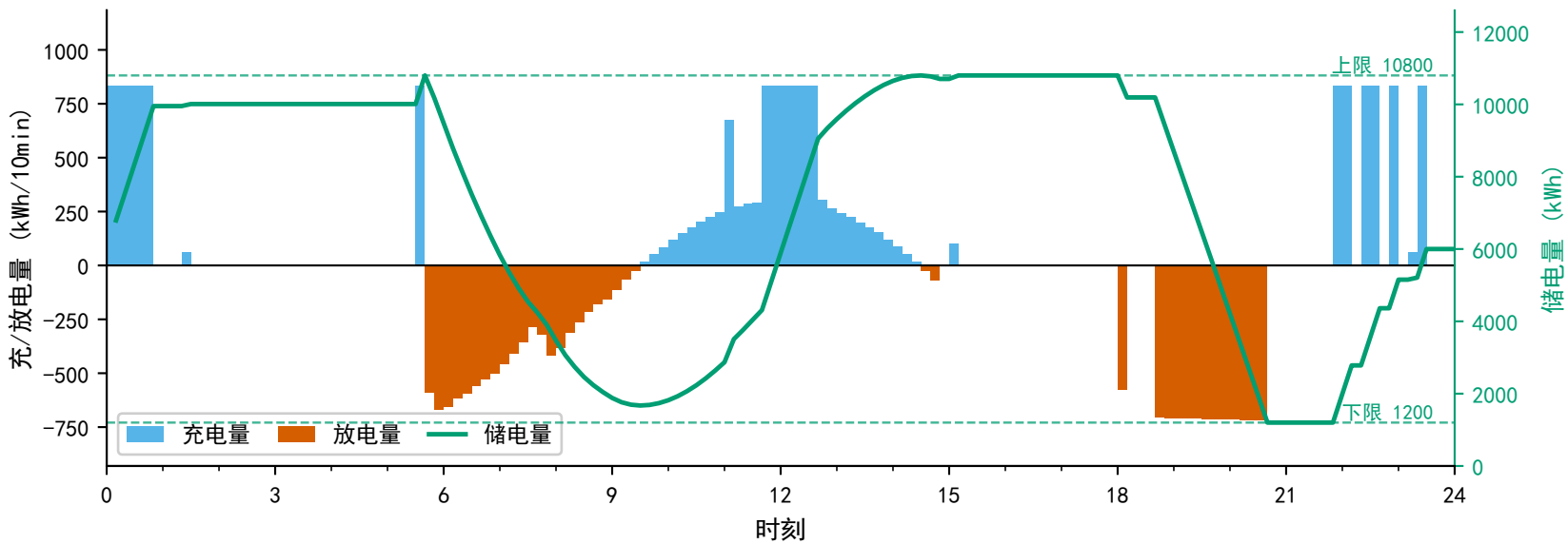
(c) 储能充放电与储电量
