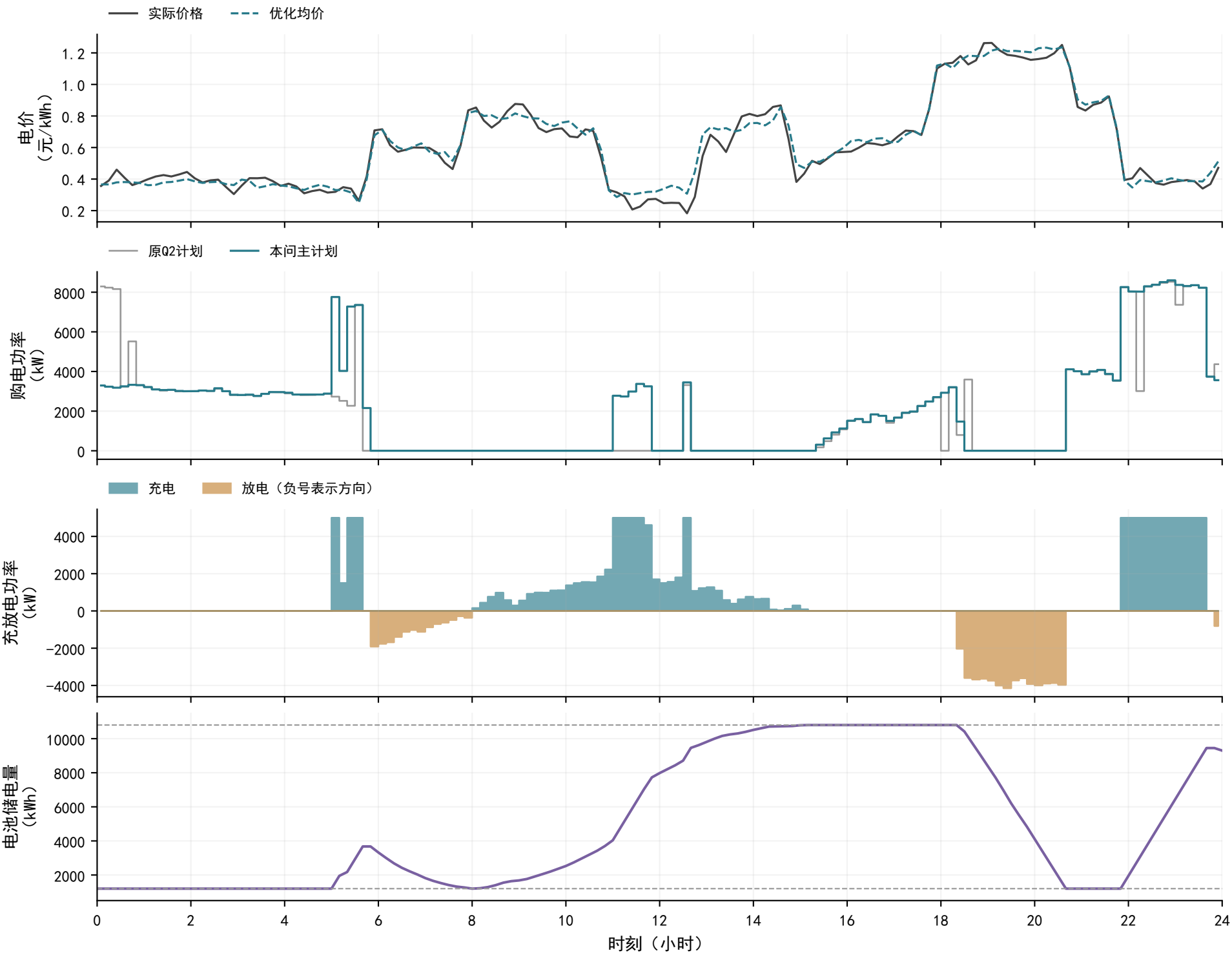
2025-06-21：波动电价下的调度
