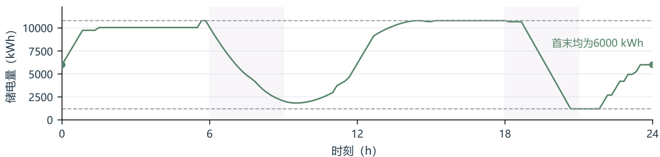
(d) 储能状态与容量边界
