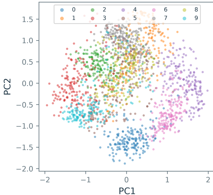
Two PCA coordinates
