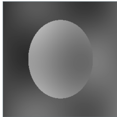
JPEG2000: 50.5 dB
