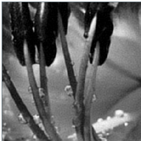
Sobolev 22.8 dB
