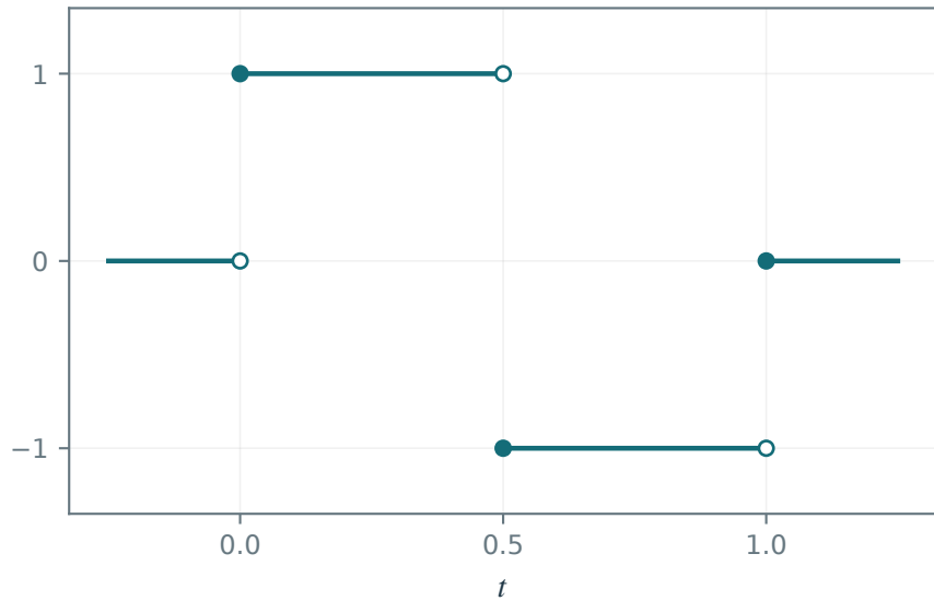
Haar wavelet \psi
