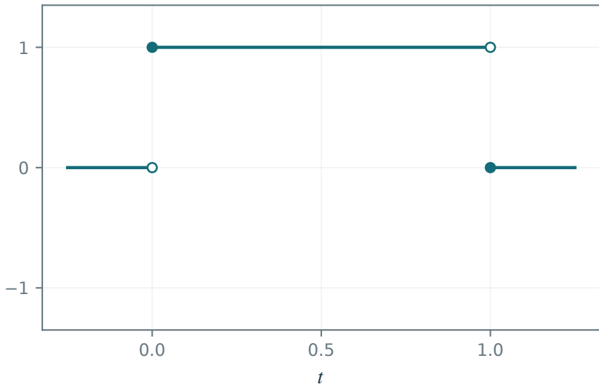
Haar scaling function \phi
