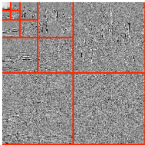
\langle f, \psi_{j,n}^\omega \rangle
