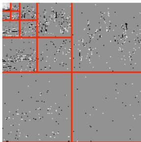
S_T(\langle f, \psi_{j,n}^\omega \rangle)
