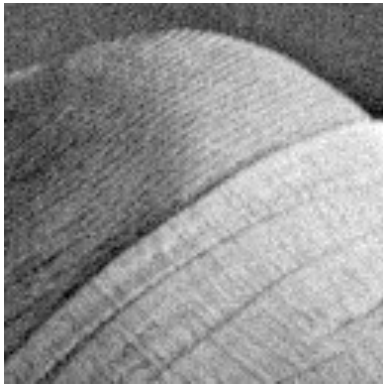
Noisy f
