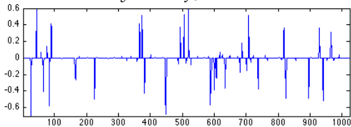
f^\star
