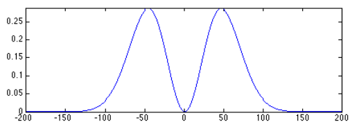
\hat{h}
