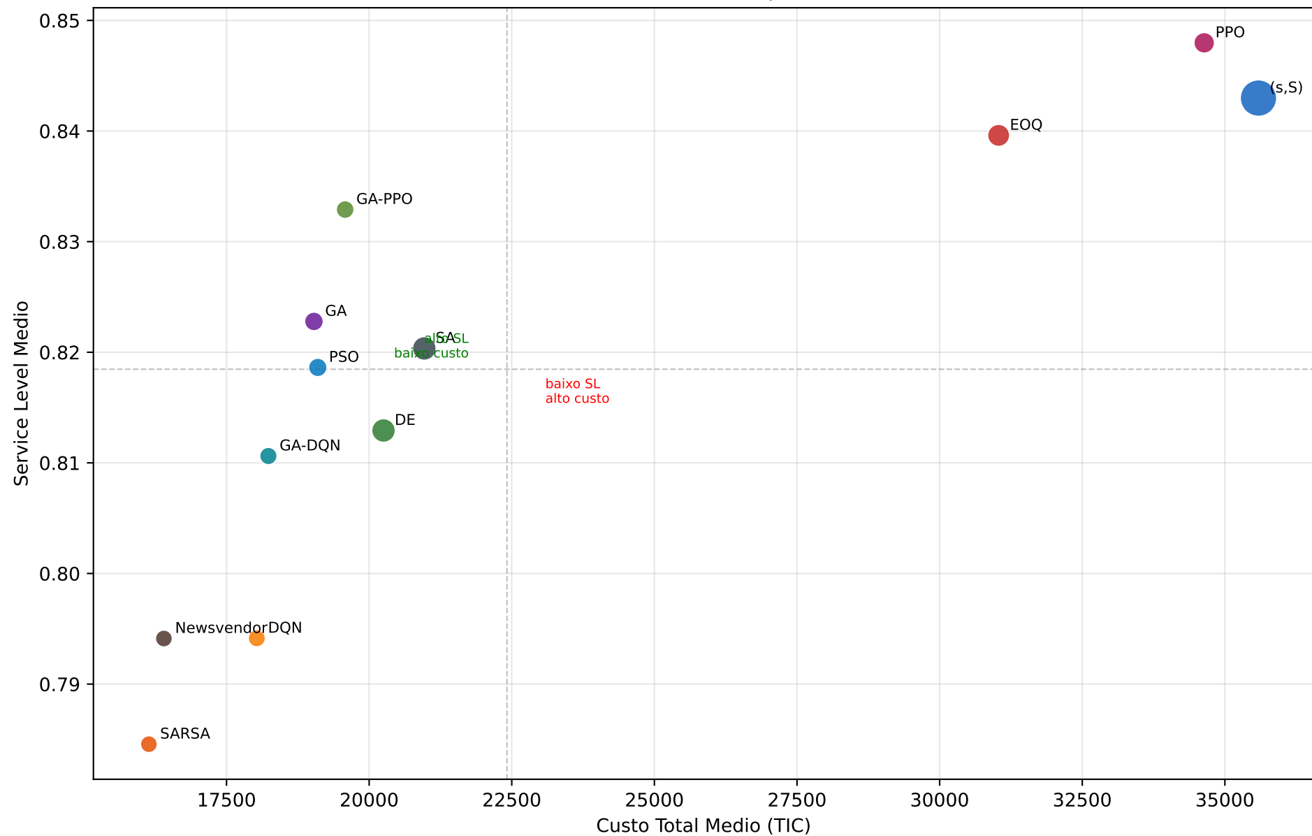
Trade-off Custo x Serviço por Política UF PB | Produto 48130 | 15 lojas (tamanho da bolha = Bullwhip Effect medio)
