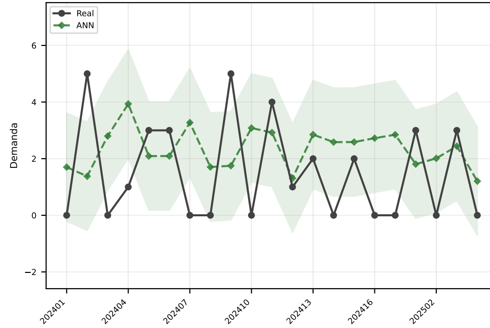
ANN MAE=1.9
