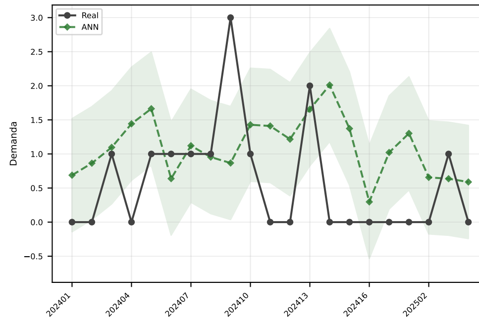
ANN MAE=0.8
