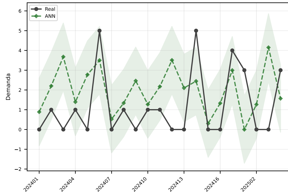
ANN MAE=1.7
