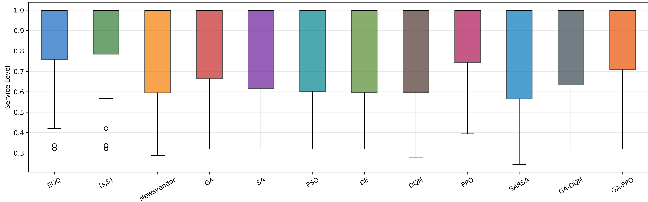
Distribuicao do Service Level por Politica — 15 Lojas UF PB | Produto 48130
