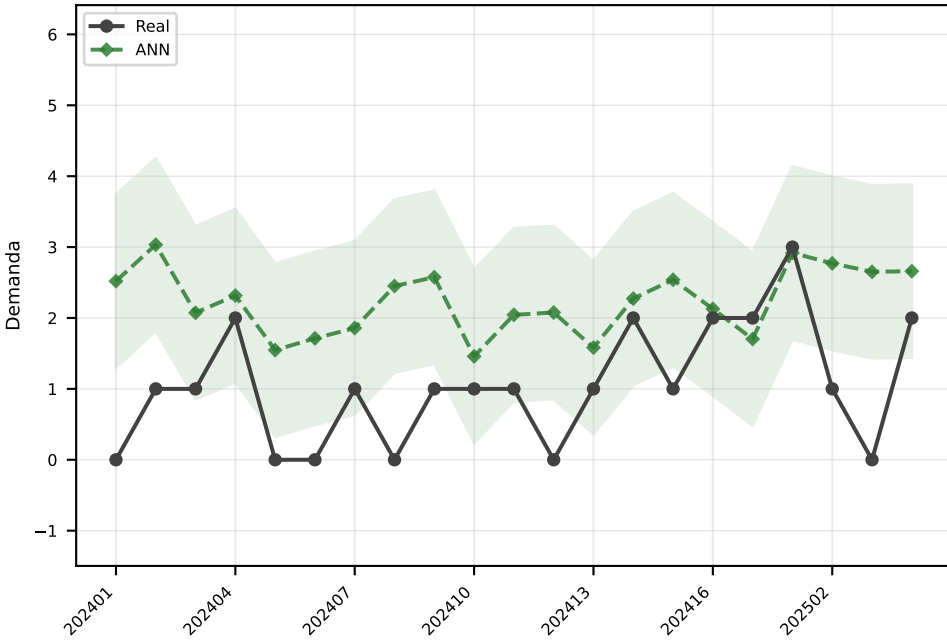
ANN MAE=1.2
