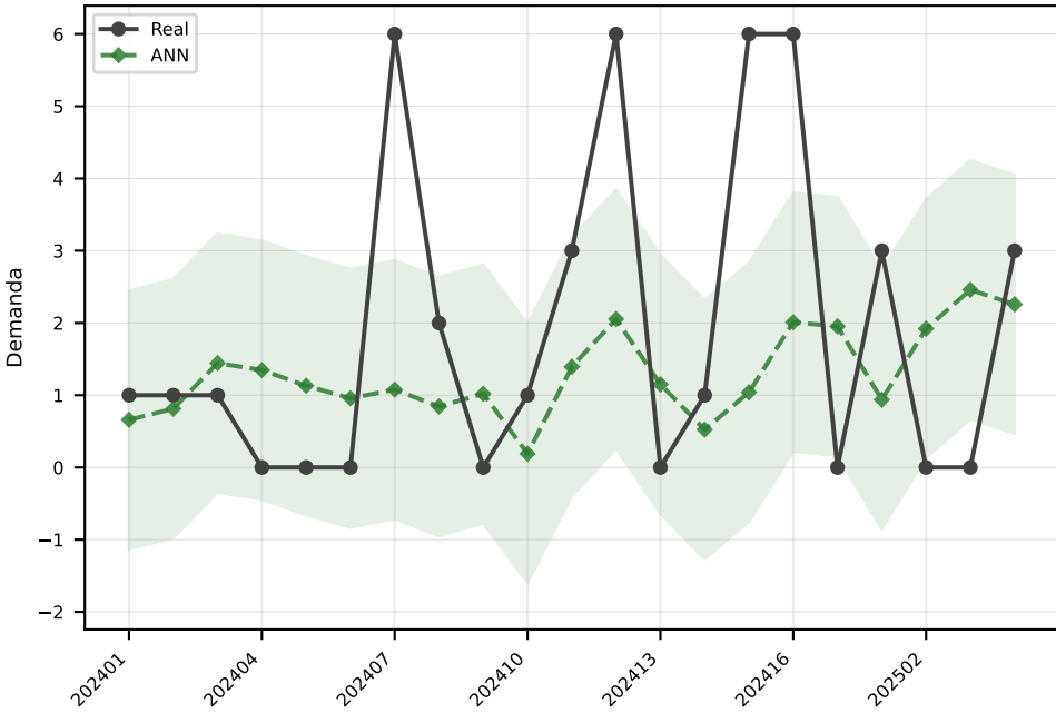
ANN MAE=1.8
