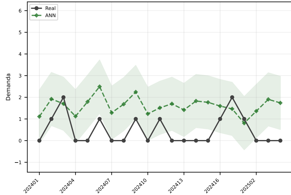
ANN MAE=1.2
