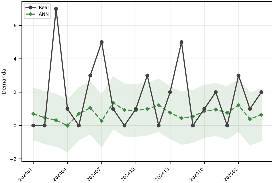
ANN MAE=1.6
