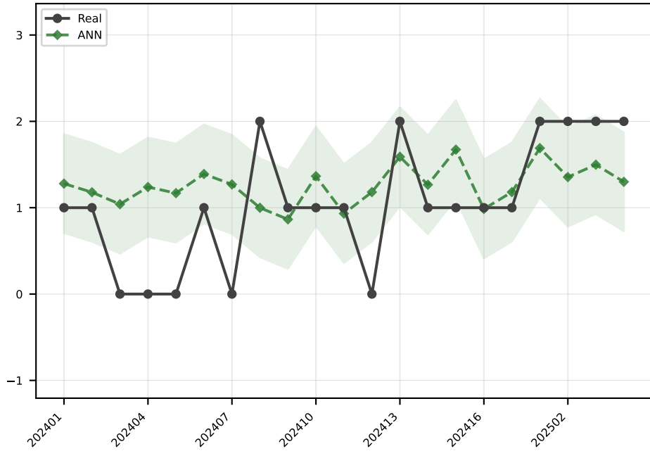
ANN MAE=0.6
