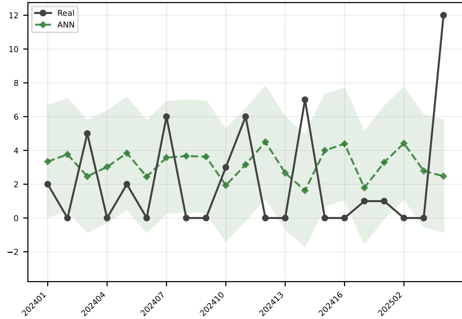
ANN MAE=3.3
